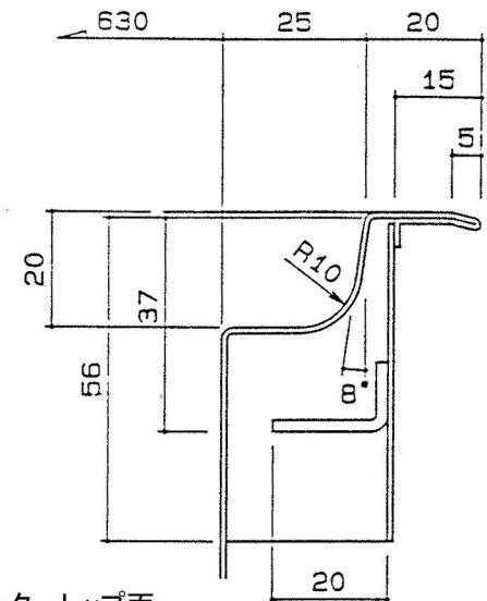
(A) 断面図
