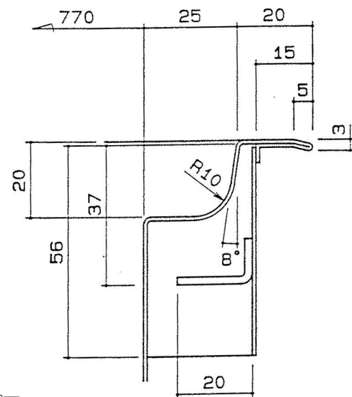
●A 断面図
